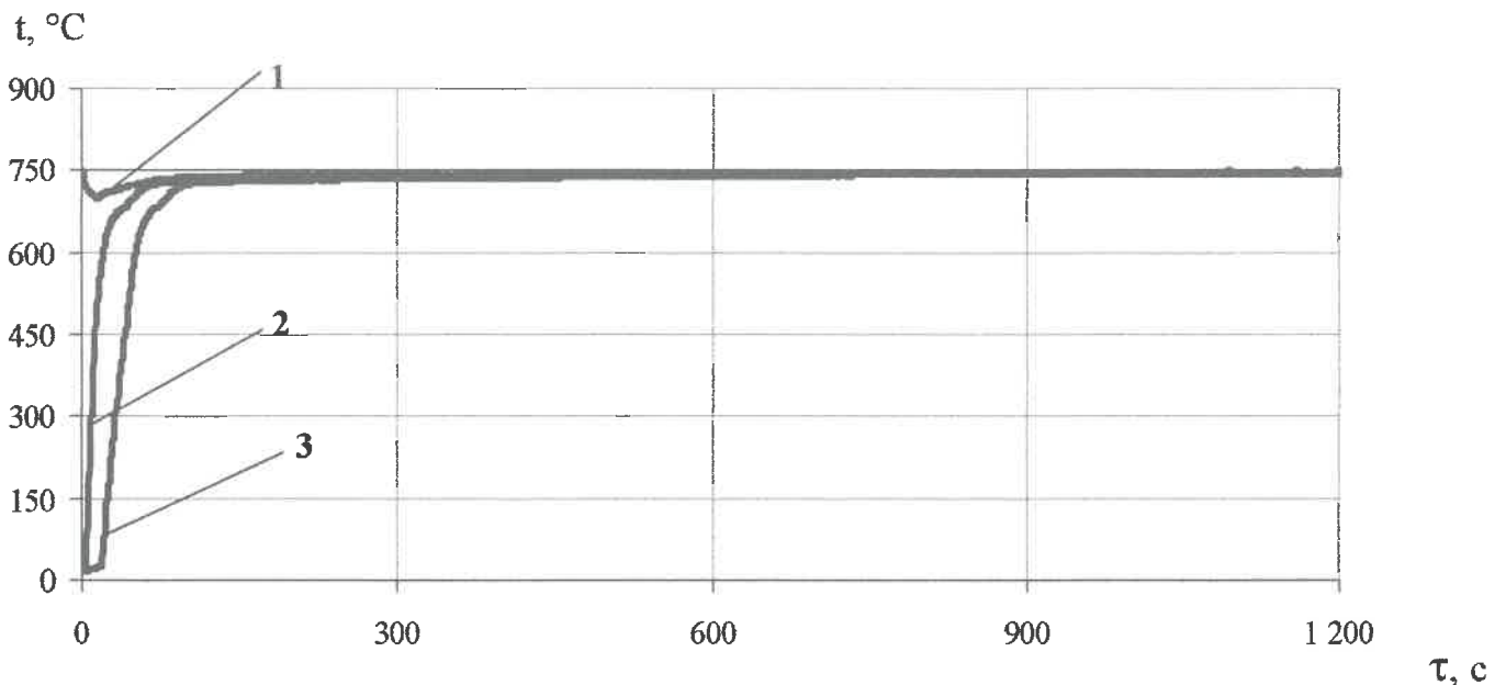
Рисунок 1 - Характерний графік змінення температури у печі (1), на поверхні (2) та всередині (3), під час випробувань зразків плити теплоізоляційної з мінеральної вати на основі скляного штапельного волокна марки «ISOVER Звукозахист», виробництва ООО "Сен-Гобен Строительная Продукция Рус".
